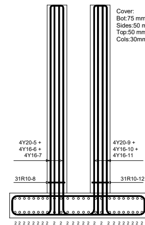
SECTION 'C-C' 1:50
