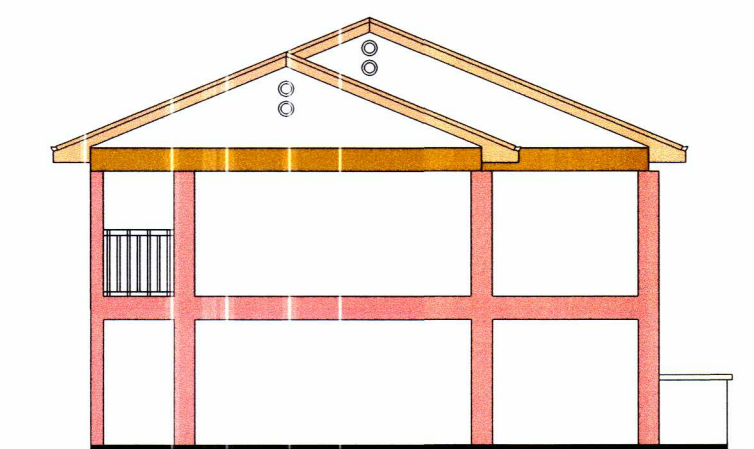
RHS ELEVATION
