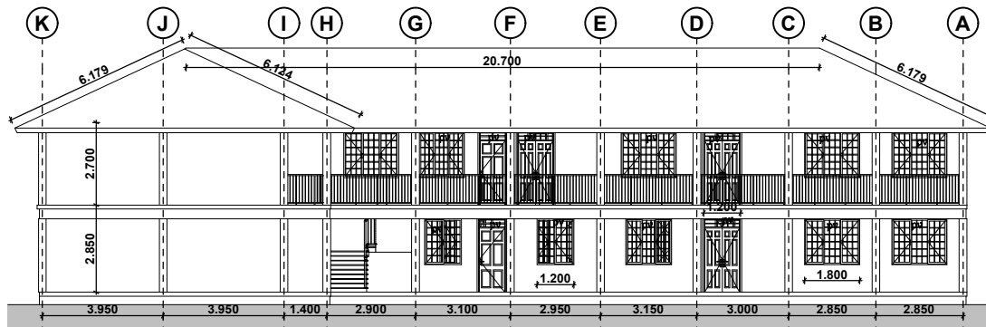
ELEVATION 04
