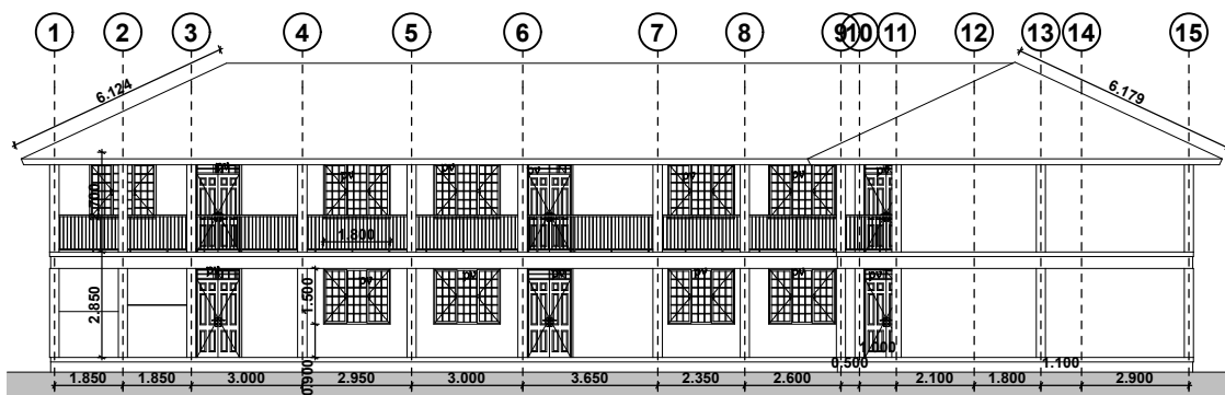
ELEVATION 01
