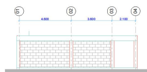
ELEVATION 04
