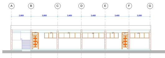
ELEVATION 01
