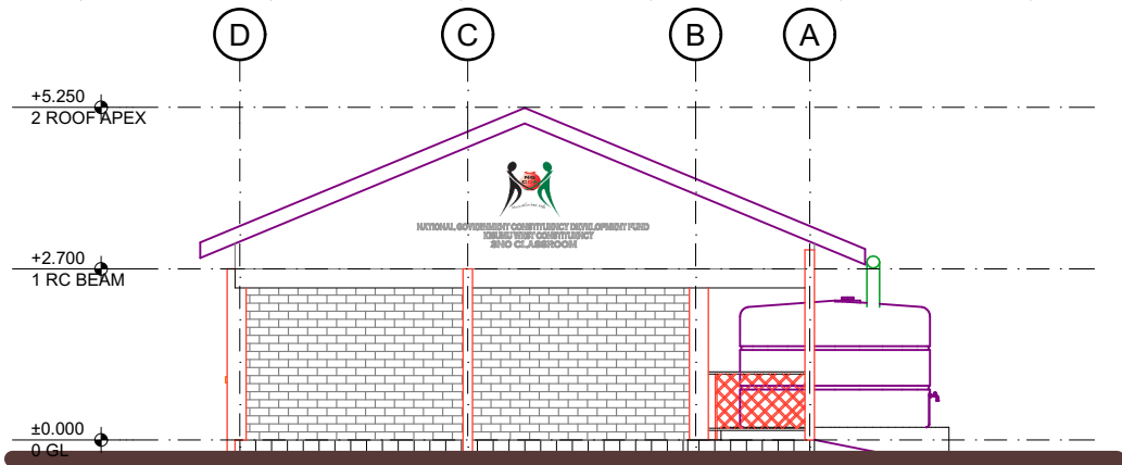
ELEVATION E-4
