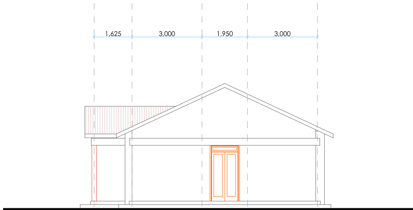
ELEVATION 02
