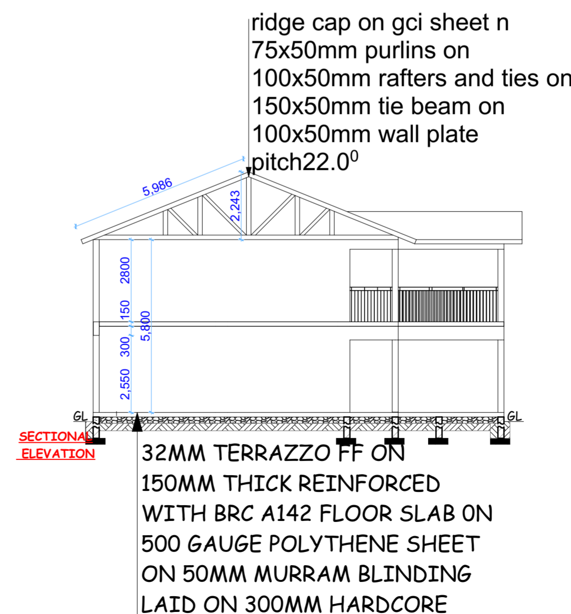
ELEVATION 04
